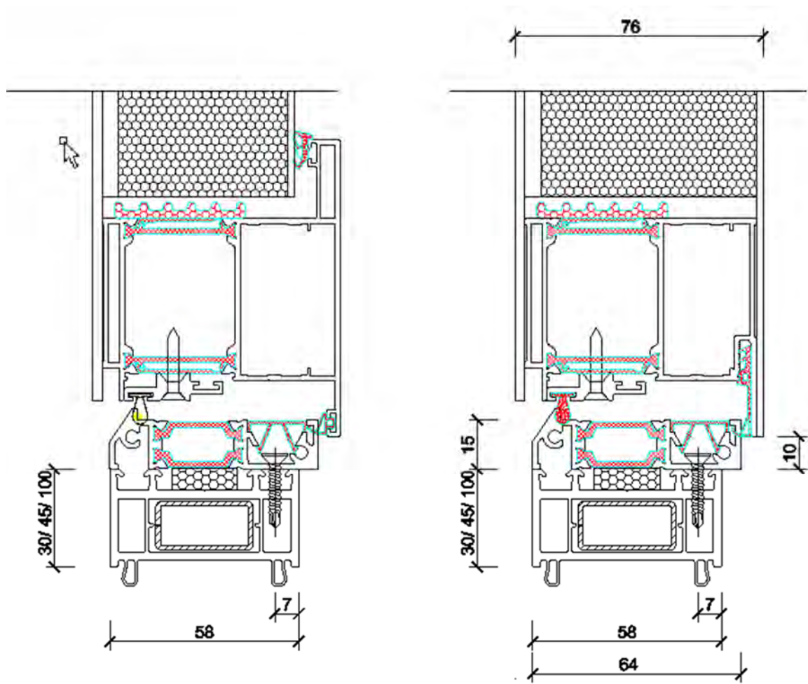
Bodeneinstandsprofil 58 mm aus Kunststoff mit Stahl – Montage unter der Schwelle
